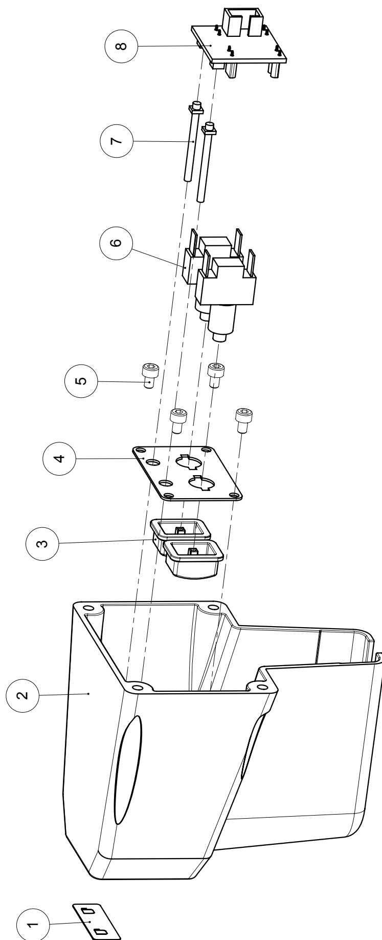
O5) COPRIMONTALATTE ASSIEME MILK FROTHER COVER ASSEMBLY
